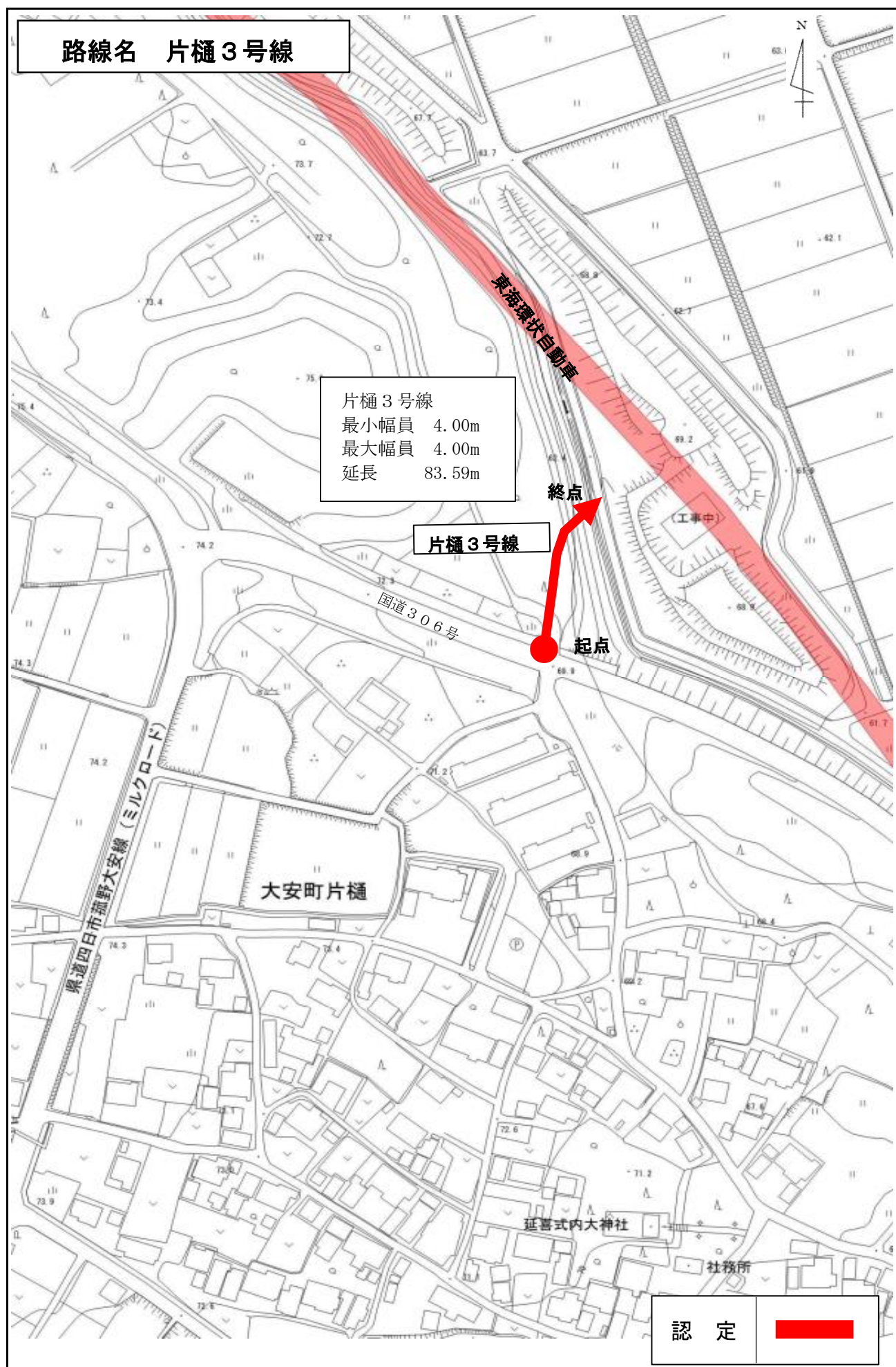
平面图
